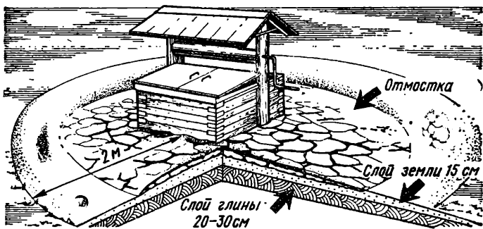
Рис. 21. Защитное оборудование колодца
